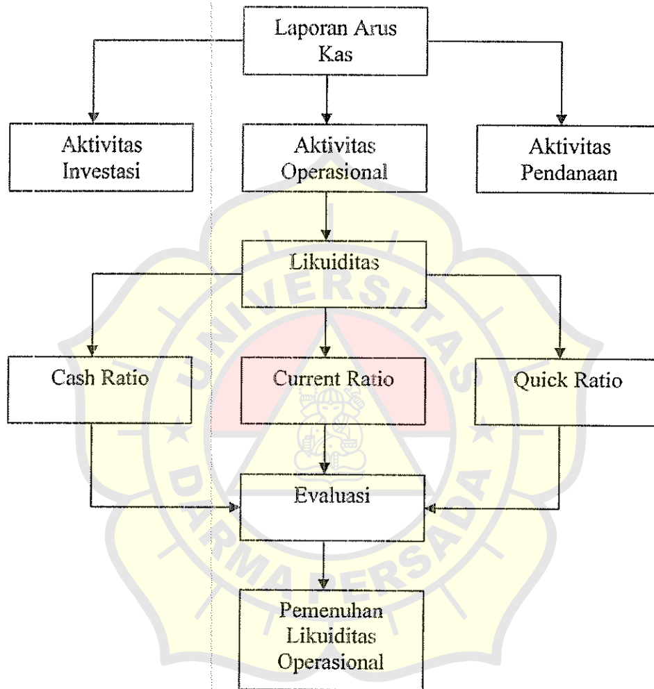
Gambar 1.1 Skema Kerangka Pemikiran
