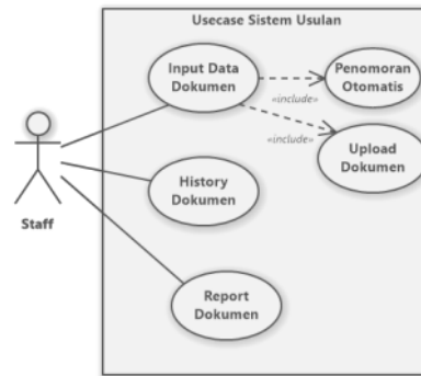
Gambar 3 Usecase Analisis Sistem Mengamen Dokumen Sistem
