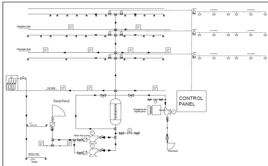
Gambar 3. Skematis sistem pemadam kebakaran
