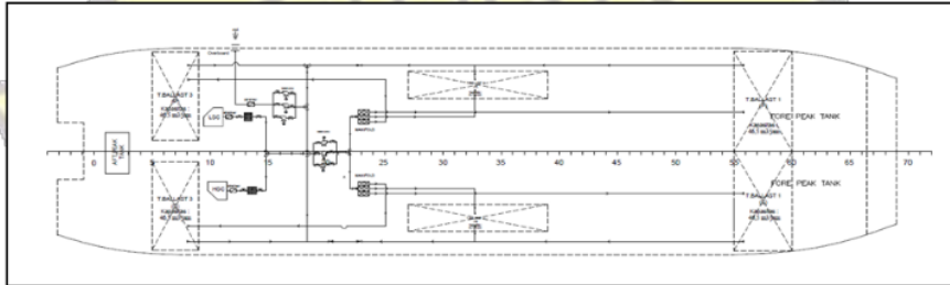
Gambar 1. Skematis sistem ballast
