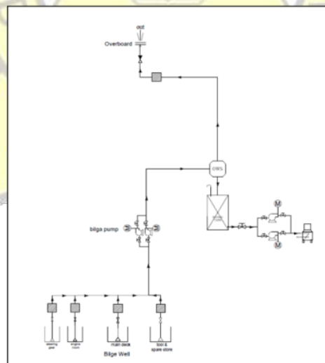
Gambar 2. Skematis sistem bilga
