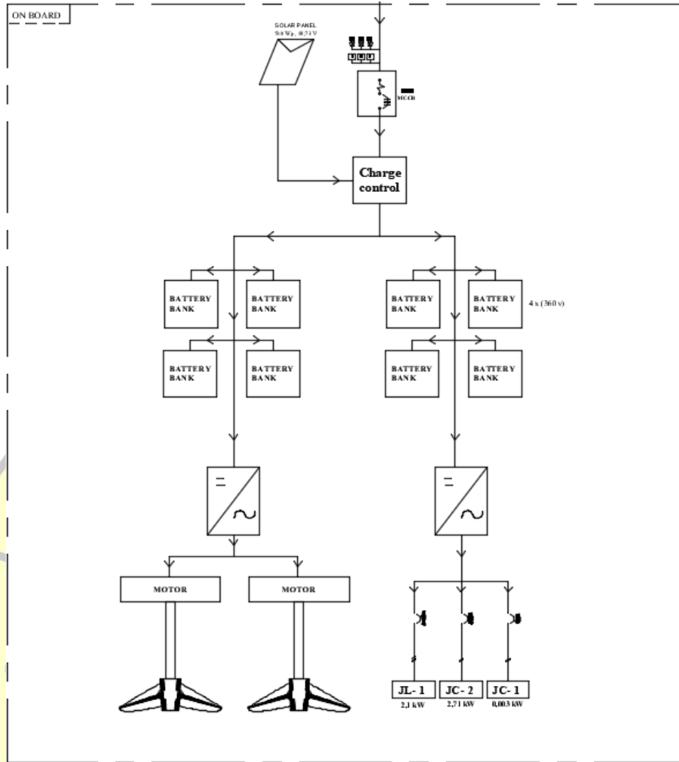
Gambar 2. Skematik Kelistrikan
