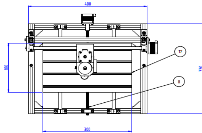
TAMPAK ATAS
