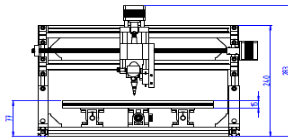
TAMPAK DEPAN
