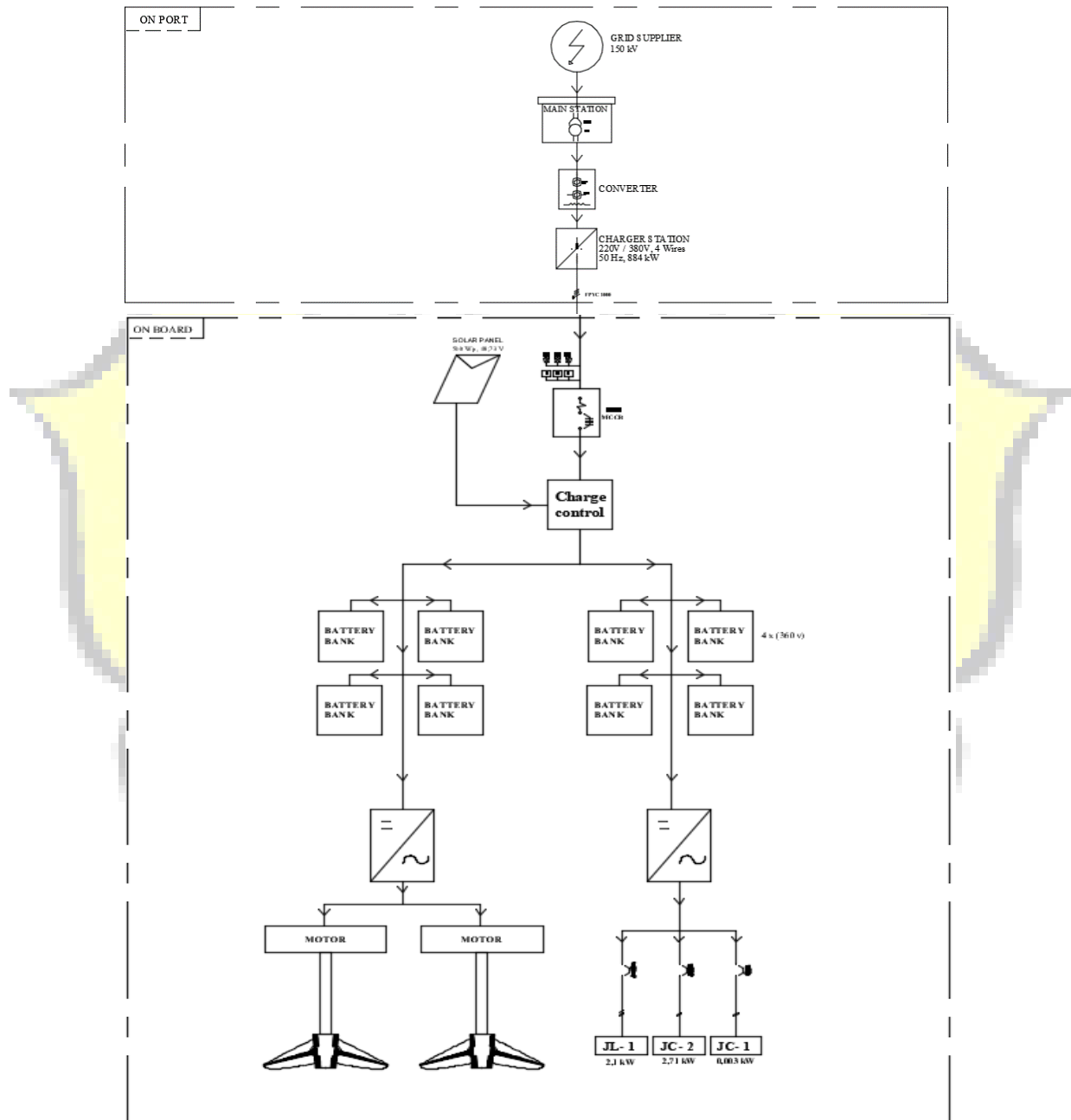
Gambar 2. Skematik Kelistrika
