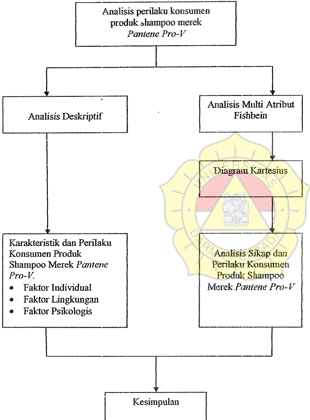
Gambar 2.1. Kerangka Skripsi
