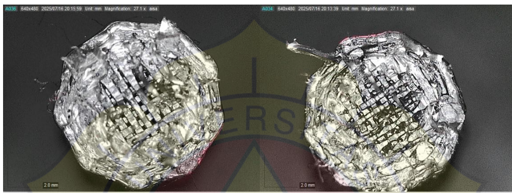
Lampiran 4. Hasil Uji Mikrostruktur Spesimen Nylon PLA 1300 RPM
